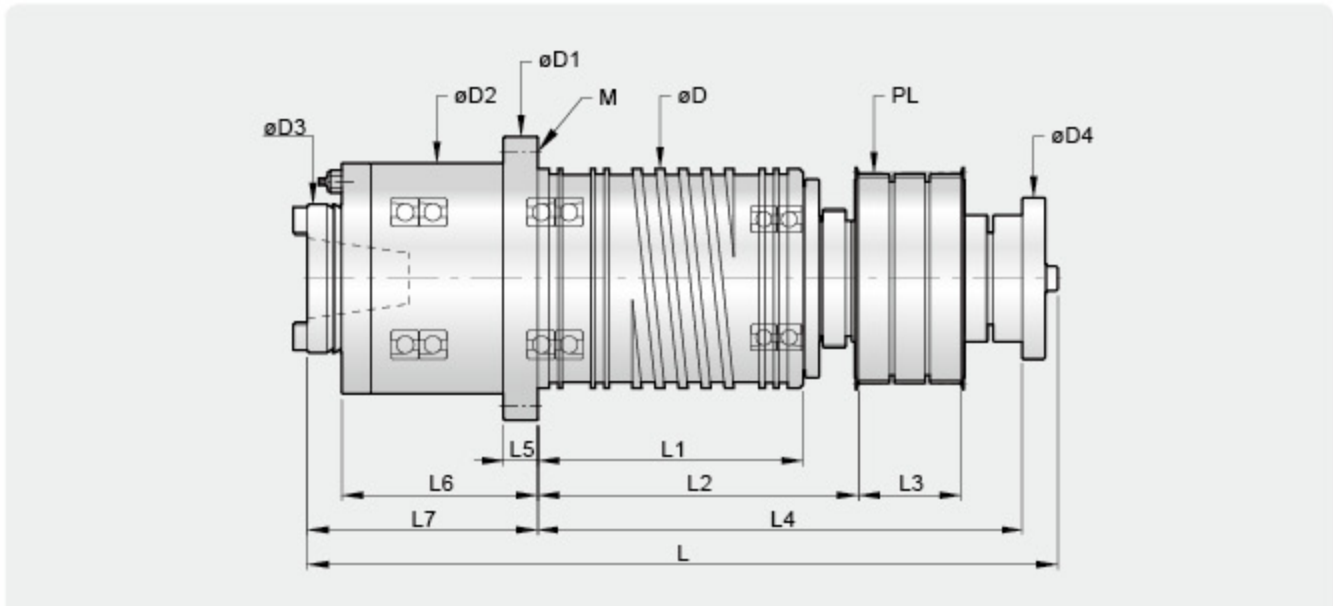
皮帶式主軸尺寸規格表
