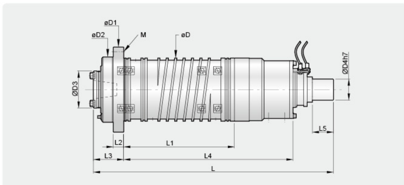
直結式主軸尺寸規格表
