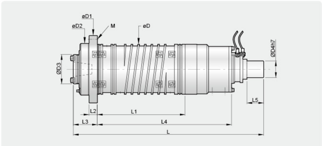
臥搪主軸尺寸規格表
